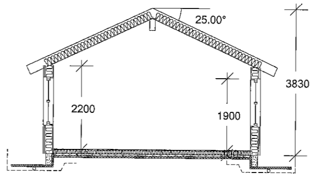
Snitt A-A
